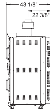
DRAFT HOOD 6" / COUPE TIRAGE 6"
